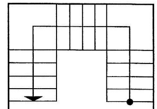
Scala a tre rampe con due curve e pianerottolo
