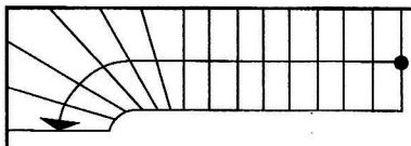
Scala ad una rampa con curva di un quarto di giro all'uscita
